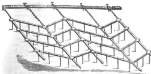
Gerrit Jan Oolman zond COLEMAN's verzet-egge in naar de tentoonstelling van de Hollandische Maatschappij van Landbouw in 1857 te Amsterdam. Door de tweede en vierde ketting langer of korter te maken, kon de afstand tussen de tanden van de egge worden ingesteld. Foto: Vriend van den Landman, 1858.
